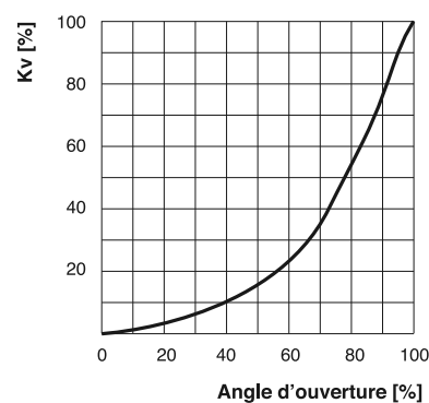
Caractéristiques de débit
