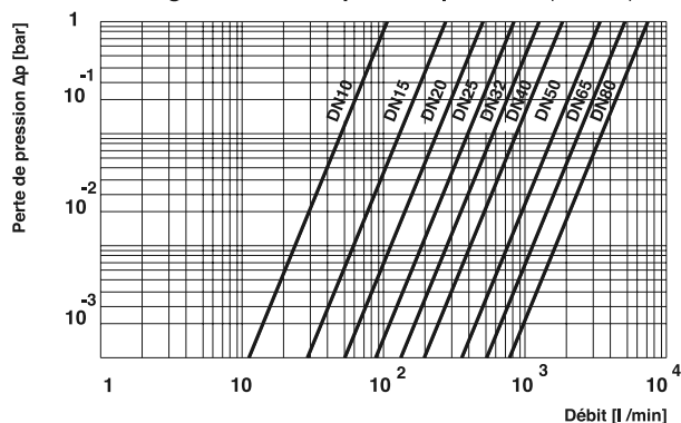
Diagramme débit / perte de pression (à 20°C)
