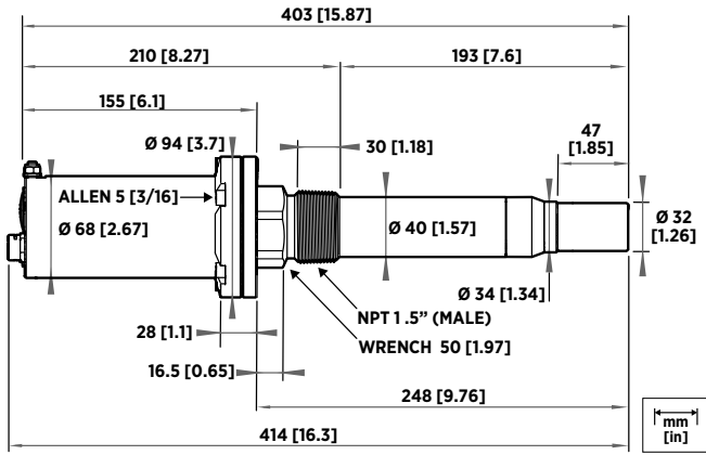
MGP261 dimensions
