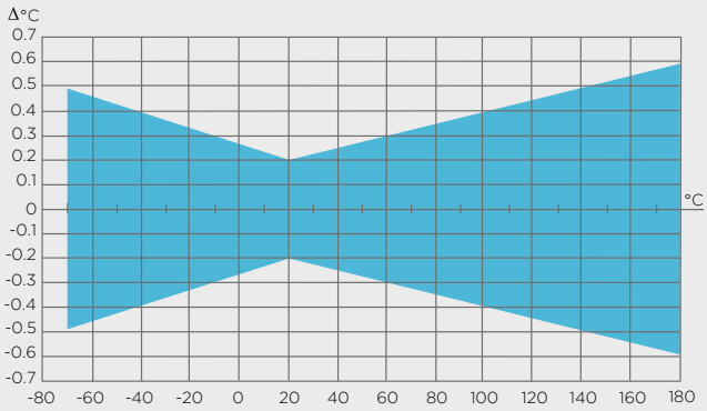
Temperature sensor Pt100 RTD Class F0.1 IEC / EN / BS EN 60751
