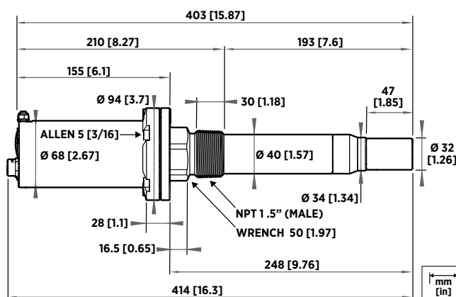
MGP262 dimensions
