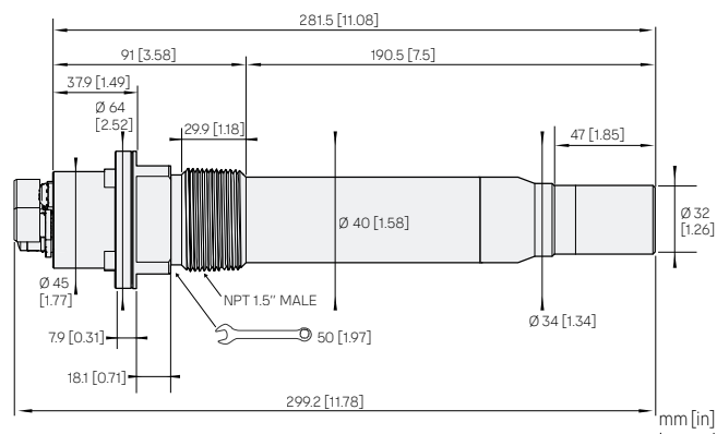
MGP241 dimensions
