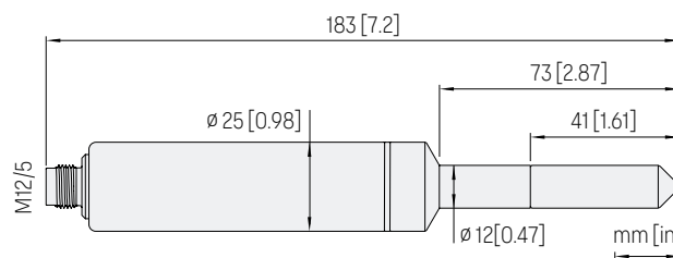
Dimensions
